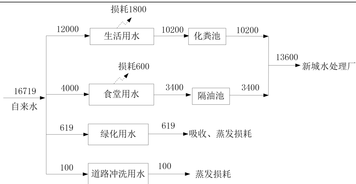
图 2-2 本次验收项目建成后实际水平衡图 单位：t/a
